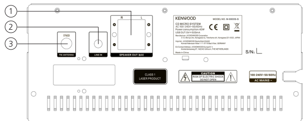
Rückseite
